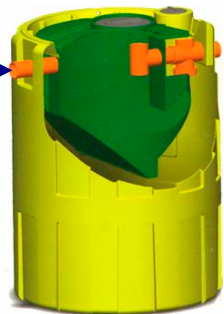
DECANTEUR-DIGESTEUR
